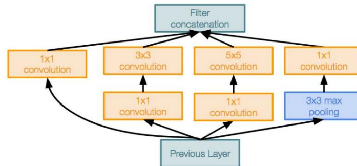
Inception module
